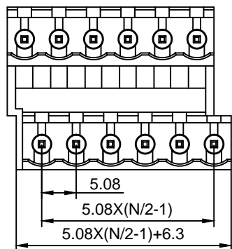
B向
